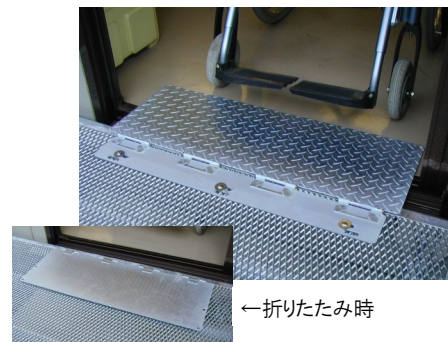
部品 サッシブリッジ700ミリ幅 アルミサッシの段差を乗り越える時に使います。 (幅700・850種類あり) 参考価格 ¥17.000-(税別、設置費別)
